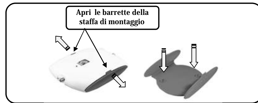
Figura 8: Montaggio a muro dell'Unità Base
